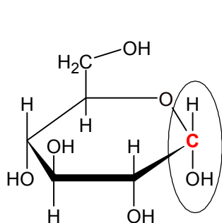
\alpha -D-Glukosa
