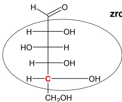
\alpha -D-Glukosa
