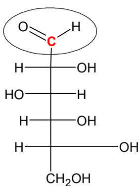
\alpha -L-Glukosa
