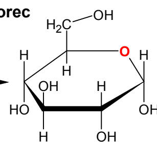
\alpha -D-Glukopyranosa
