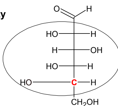
\alpha -L-Glukosa
