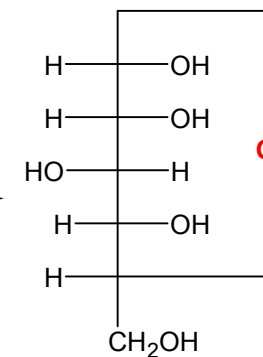
\alpha -D-Glukopyranosa
