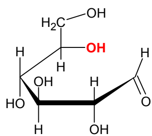
\alpha -D-Glukosa
