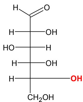
\alpha -D-Glukosa
